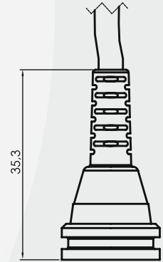
Kabelausgang (IP67) mit Knickschutz
